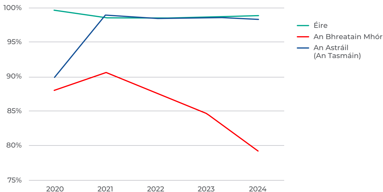
Fíor 6: Cion ama a shuíonn SF laistigh de 50 \pm 0.1 Hz (%), 2020-24
