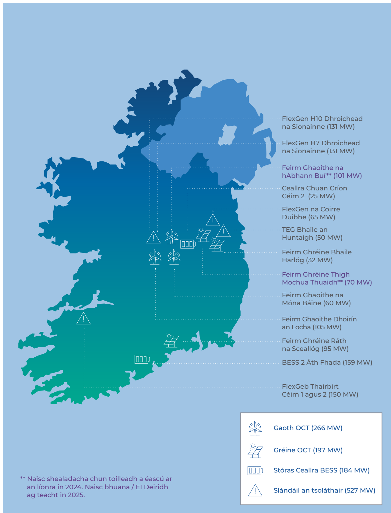
Fíor 3: Fuinnmhithe giniúna 2024
