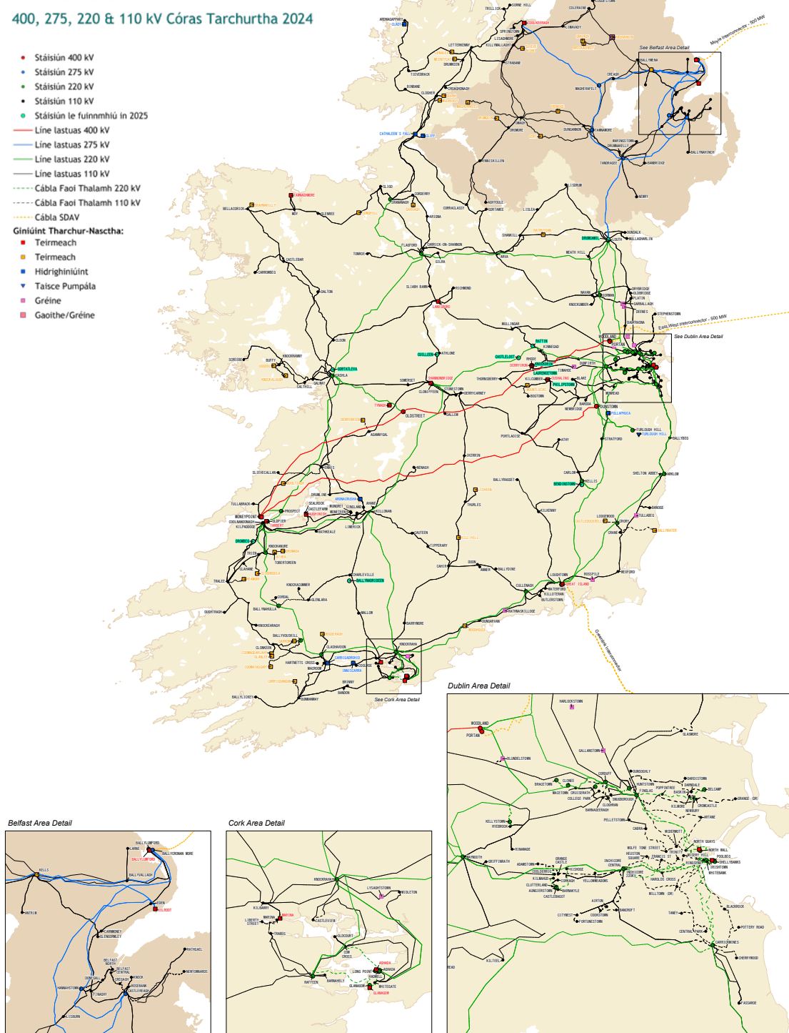
Fíor 1: Léarscáil den Chóras Tarchurtha ar fud na hÉireann 2024 10
