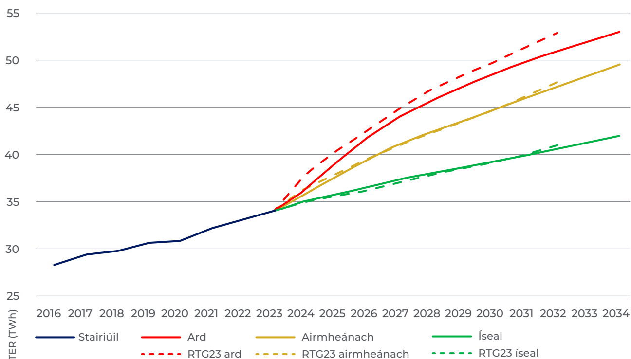
Fíor 5: Réamhaisnéis an cheanglais leictreachais iomláin d'Éirinn 2025-2034.
